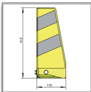
EAS-1020 hoek bescherming met bevestigingsbeugel naar binnen
