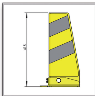
EAS-1010 hoek bescherming met bevestigingsbeugel naar buiten
